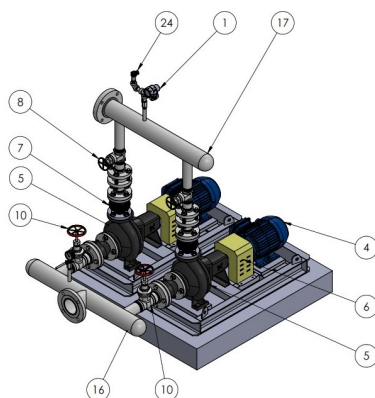
Sistema de bombeo para recirculación de agua helada para Chiller - Nexa Resourse Cajamarquilla
